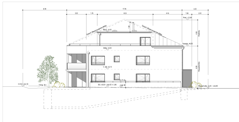
SÜDOSTFASSADE
