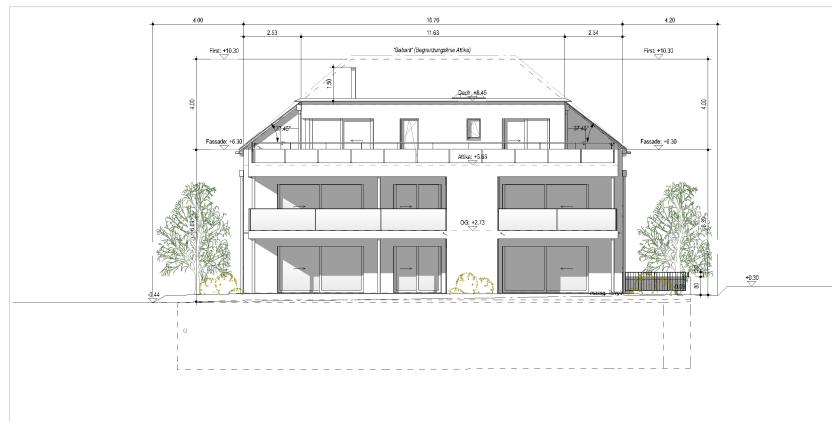
SÜDWESTFASSADE
