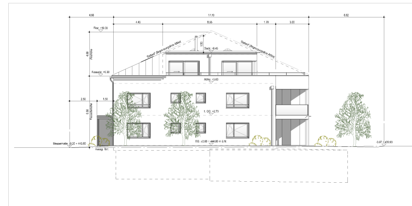
NORDWESTFASSADE
