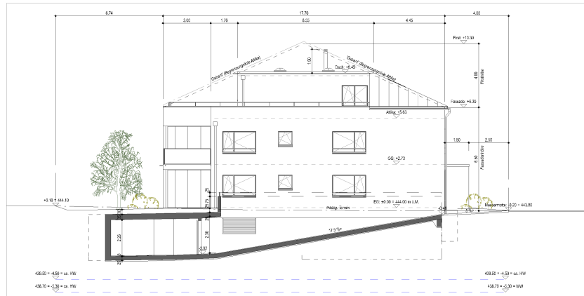
QUERSCHNITT C-D
