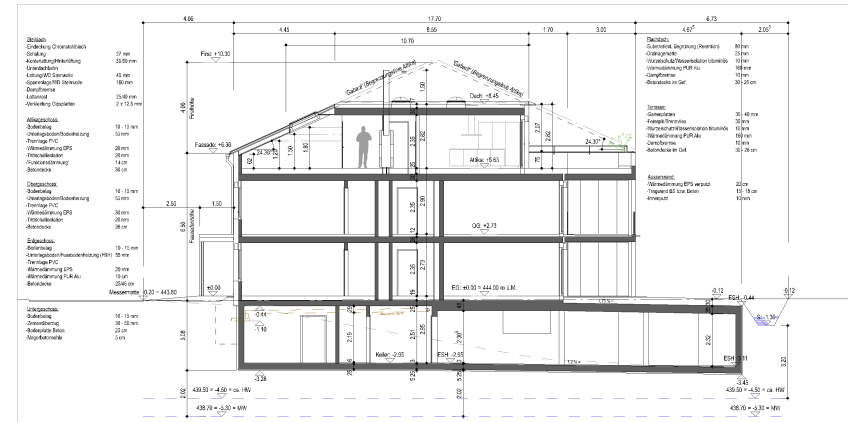
QUERSCHNITT A-B
