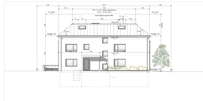
NORDOSTFASSADE
