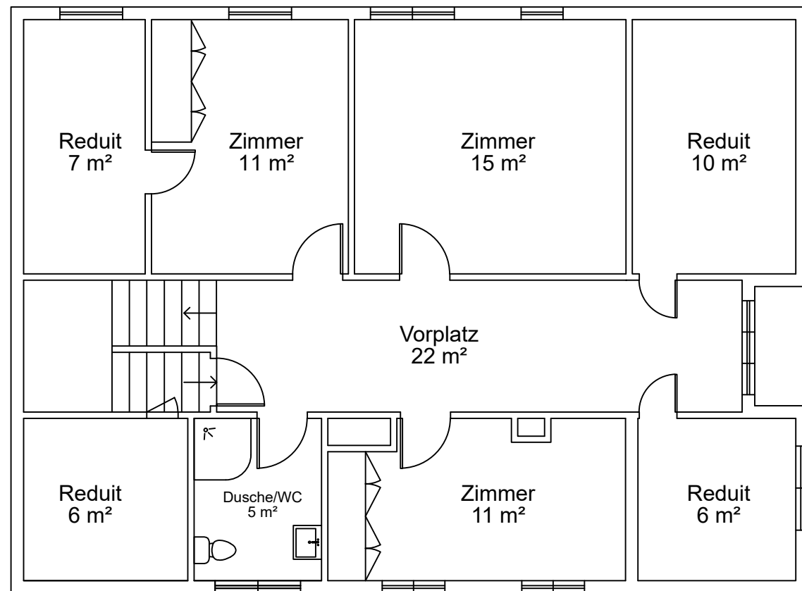
OBERGESCHOSS
