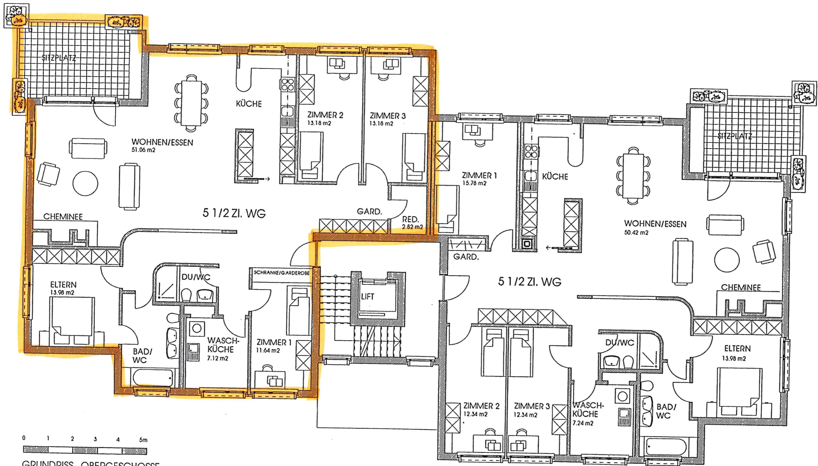
GRUNDRISS OBERGESCHOSSE
