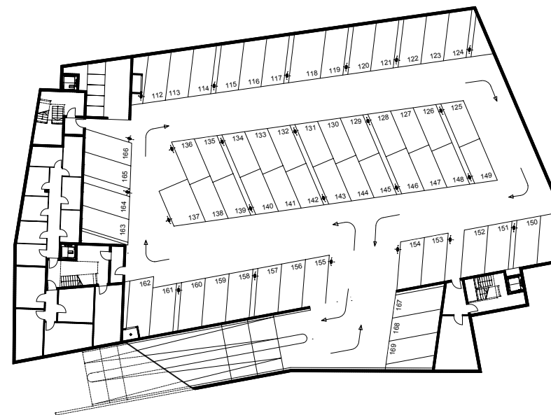
2. Untergeschoss: 58 Parkplätze
