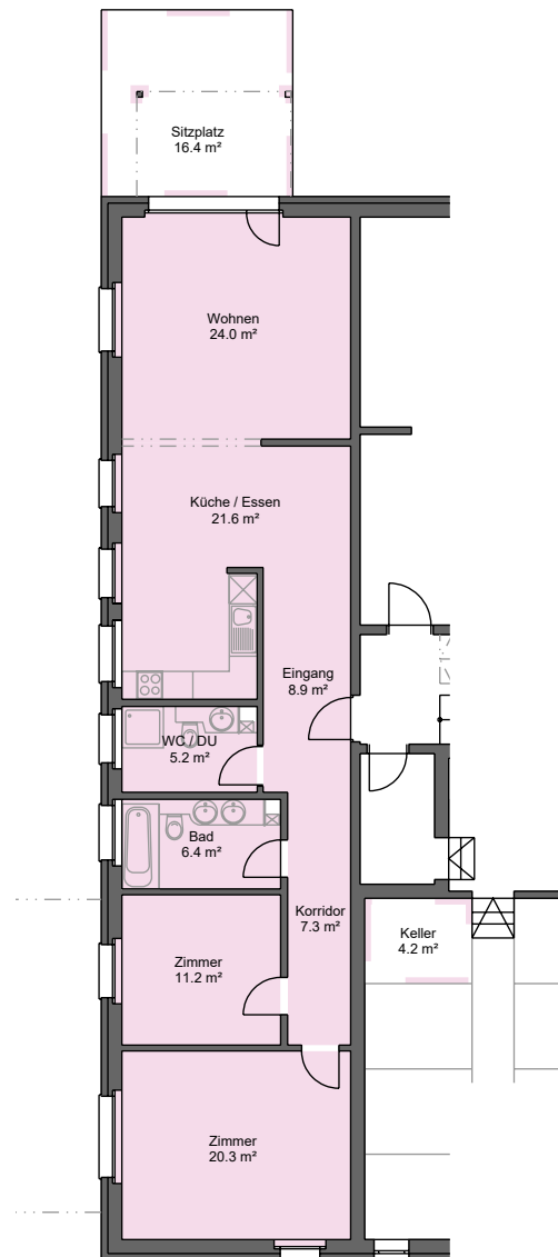
Erdgeschoss
