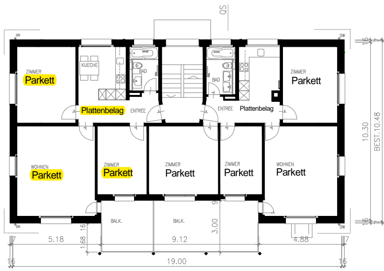
ERDGESCHOSS – 2.OBERGESCHOSS
