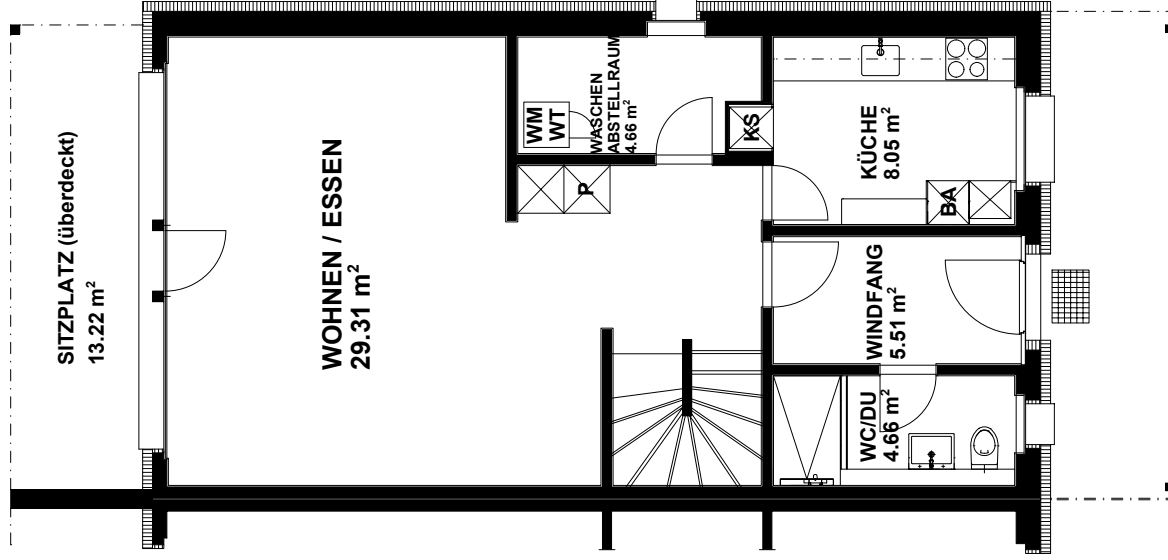
Erdgeschoss 1:100
