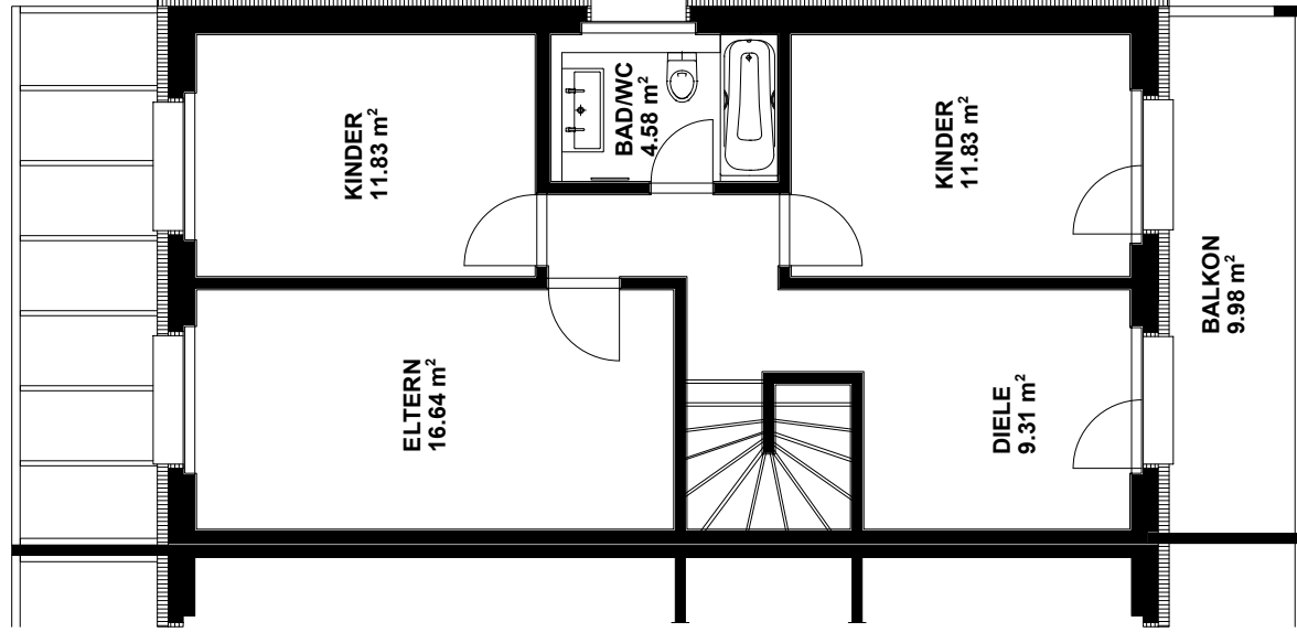
Obergeschoss 1:100
