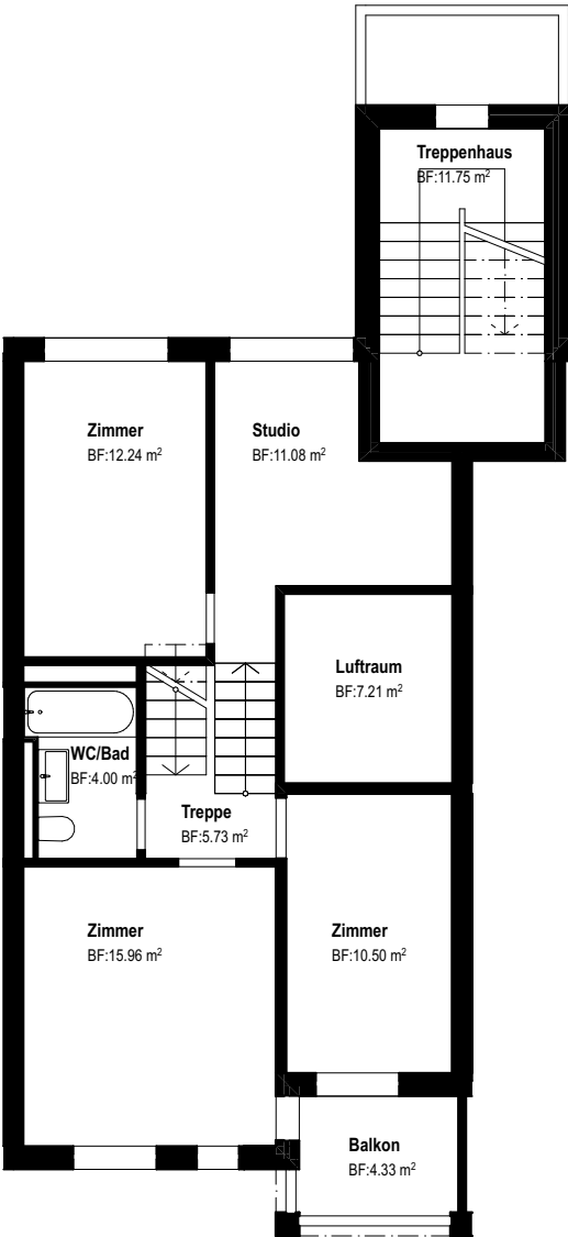
1. Obergeschoss 1:125
