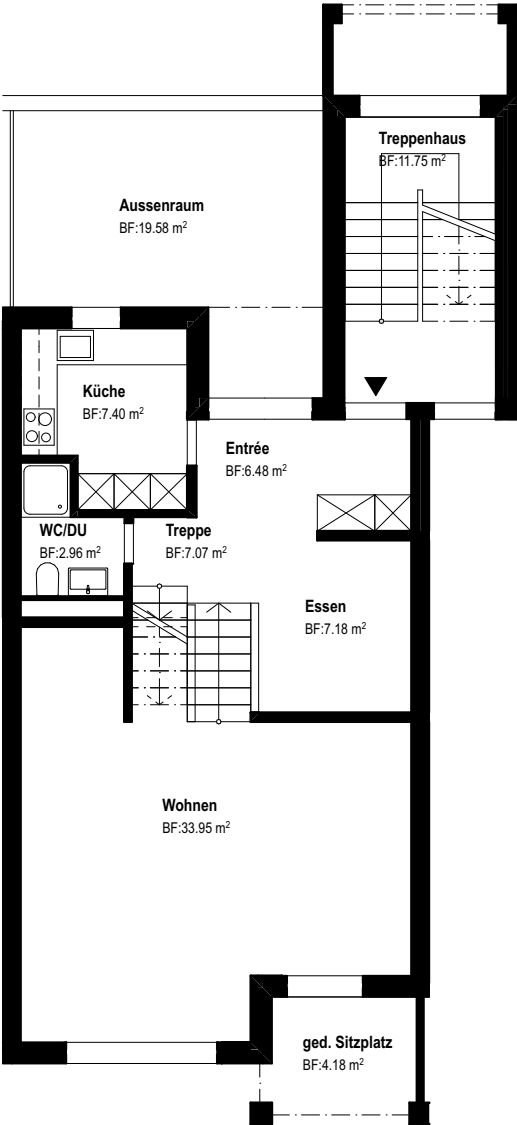
Erdgeschoss 1:125
