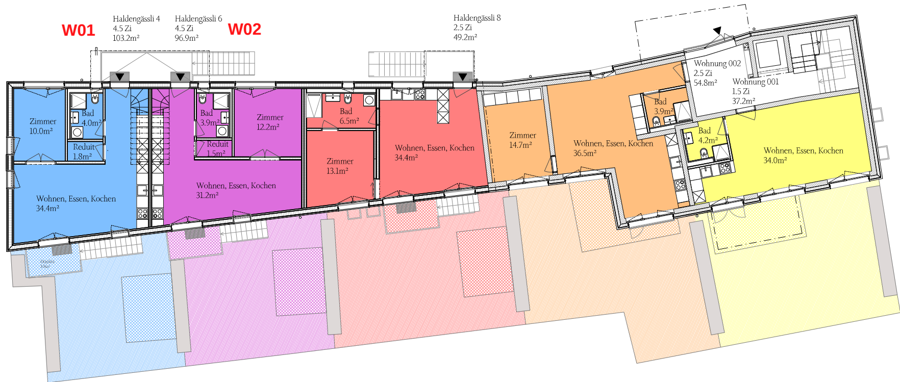
Grundriss 0. Erdgeschoss
