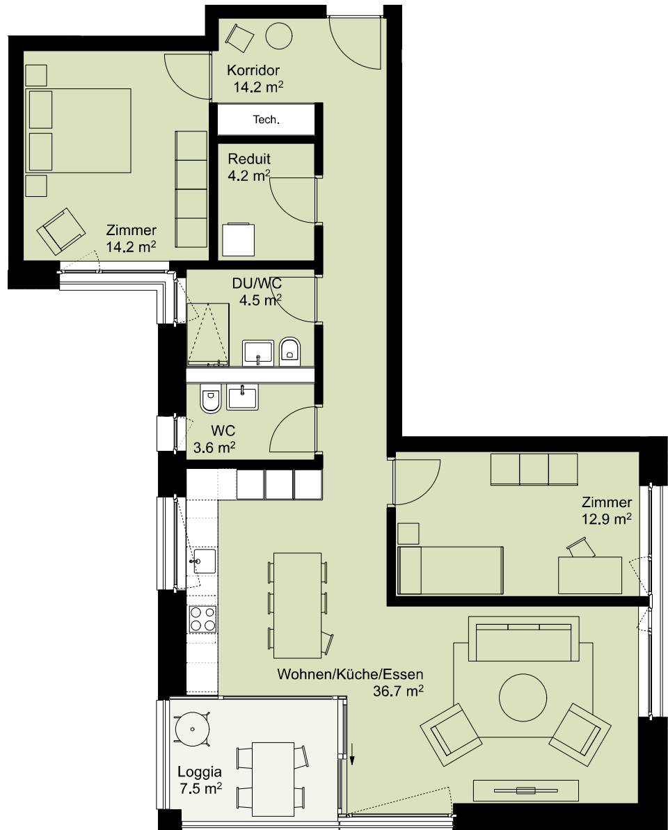
Grundriss 1. Obergeschoss 1:100
