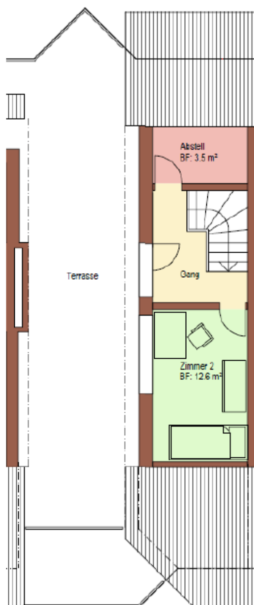
Wohnungstyp W13 3.5 Zimmer Wohnung ca. 86 m 2 Nr. 2, 5, 16, 19
