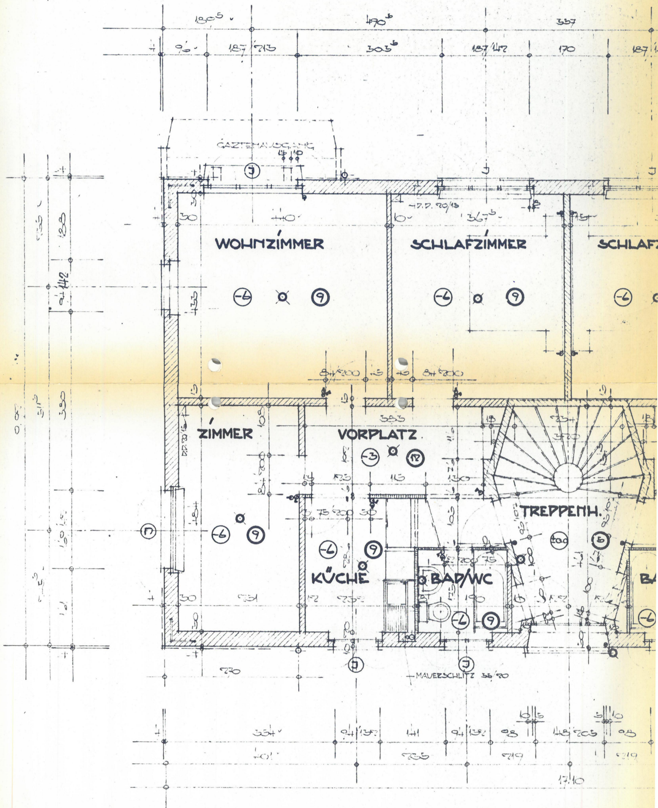
ERDGESCHOSS
