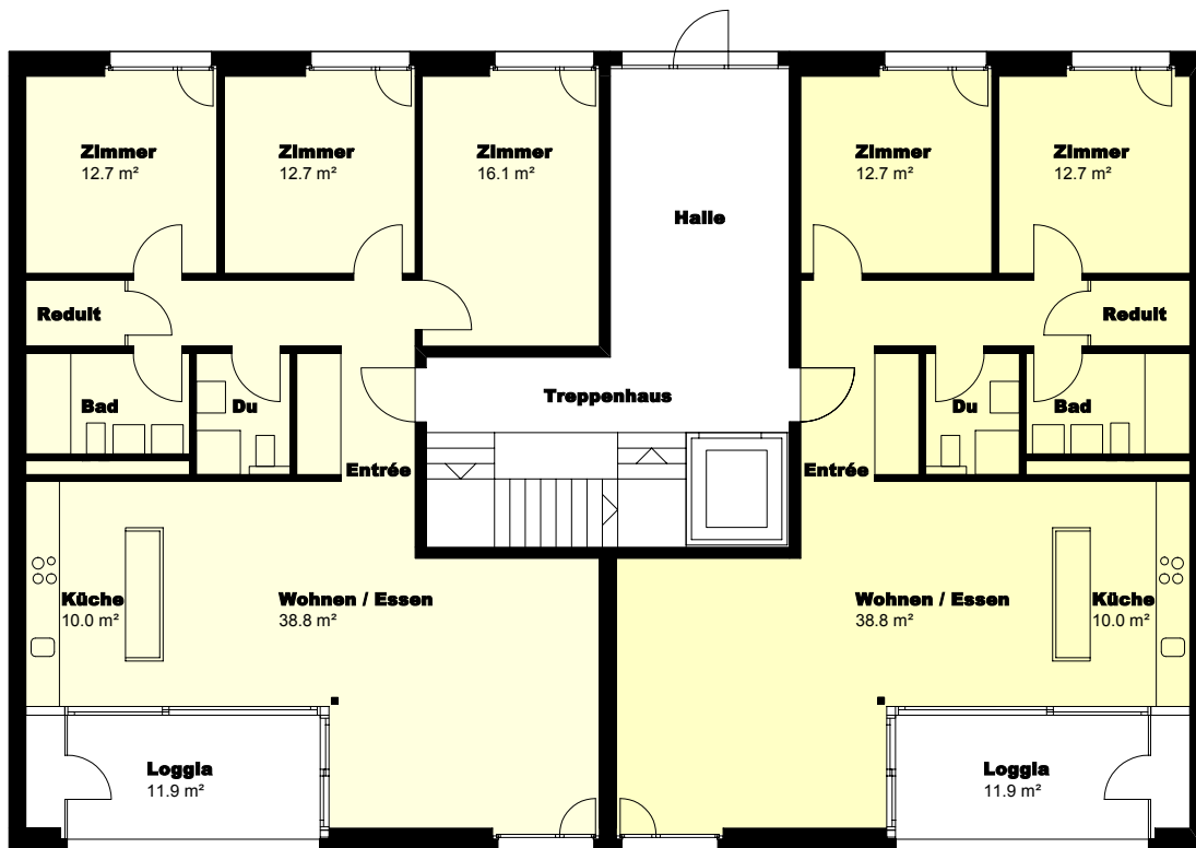
Grundriss M. 1:150
