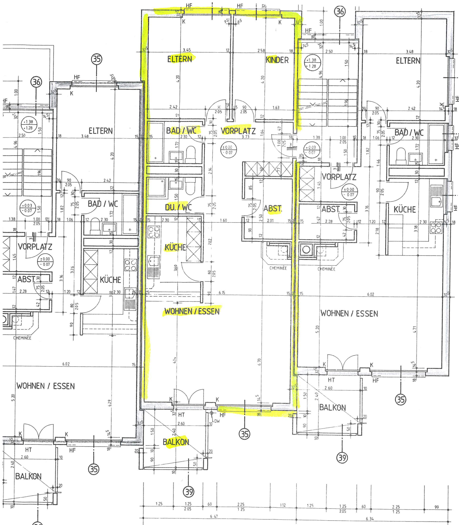
HAUS C 2. OBERGESCHOSS
