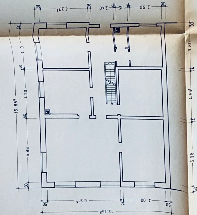
GRUNDRISS 1. OBERGESCHOSS
