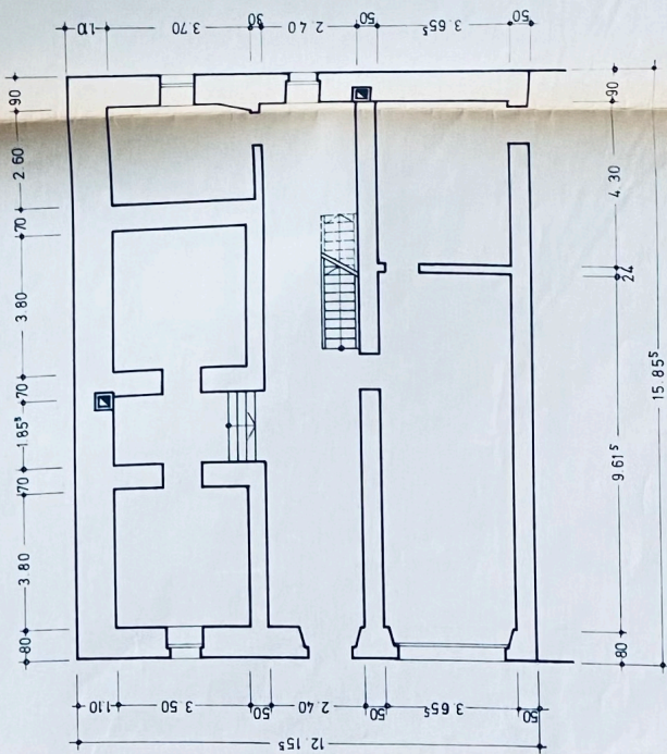
GRUNDRISS ERD- UND KELLERGESCHOSS
