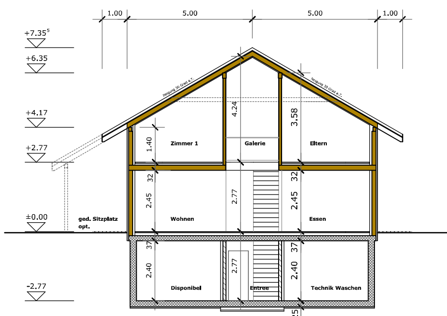
Querschnitt
