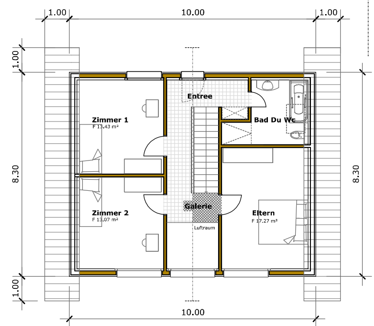
Obergeschoss
