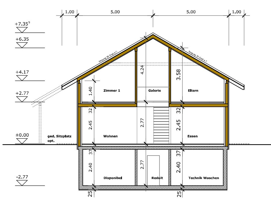
Querschnitt
