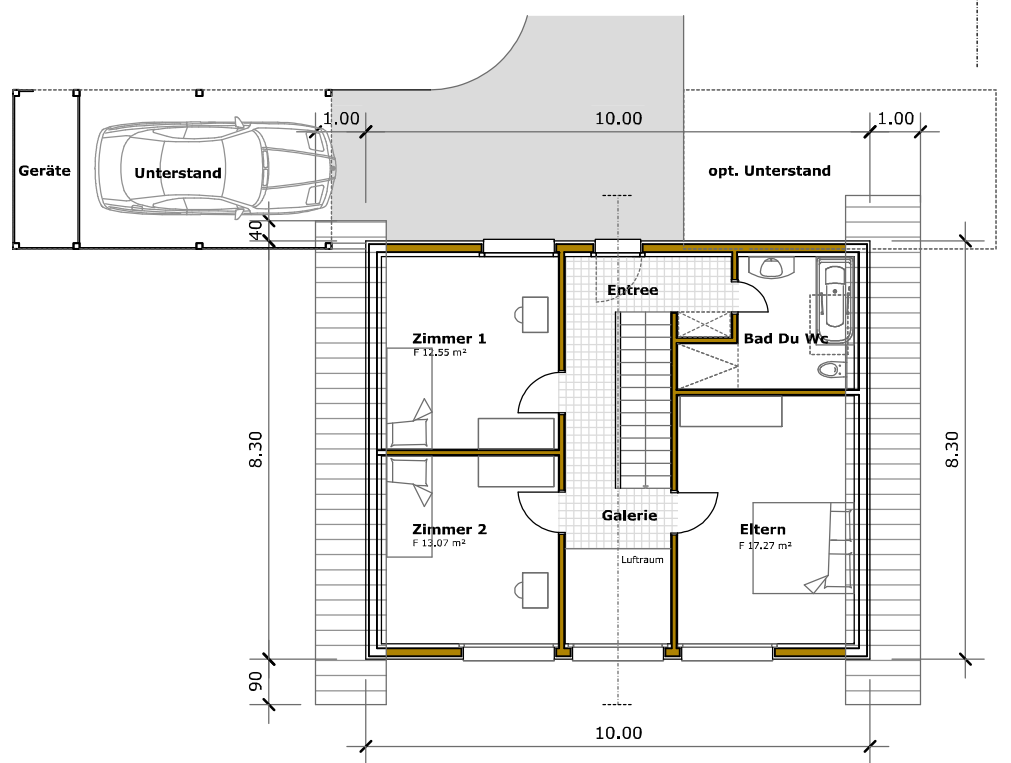
Obergeschoss
