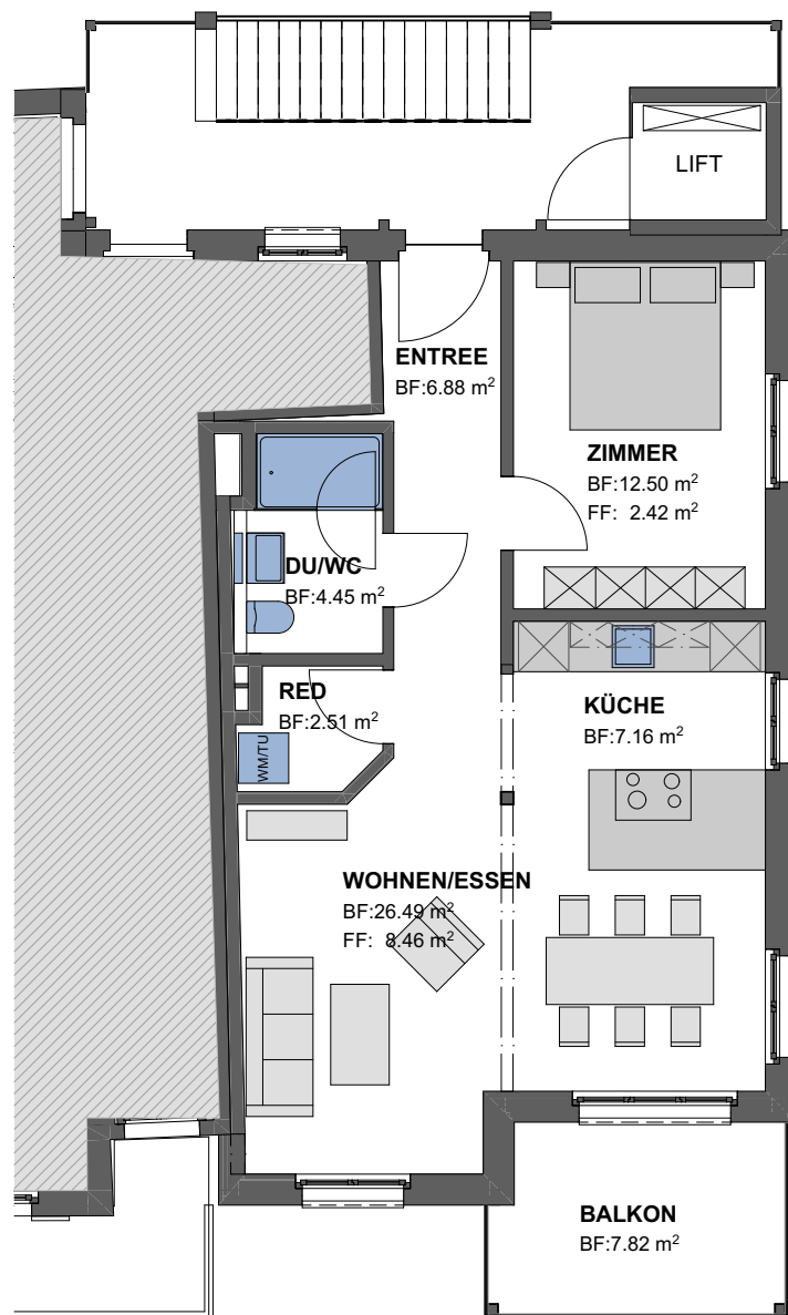
GRUNDRISS1 OBERGESCHOSS
