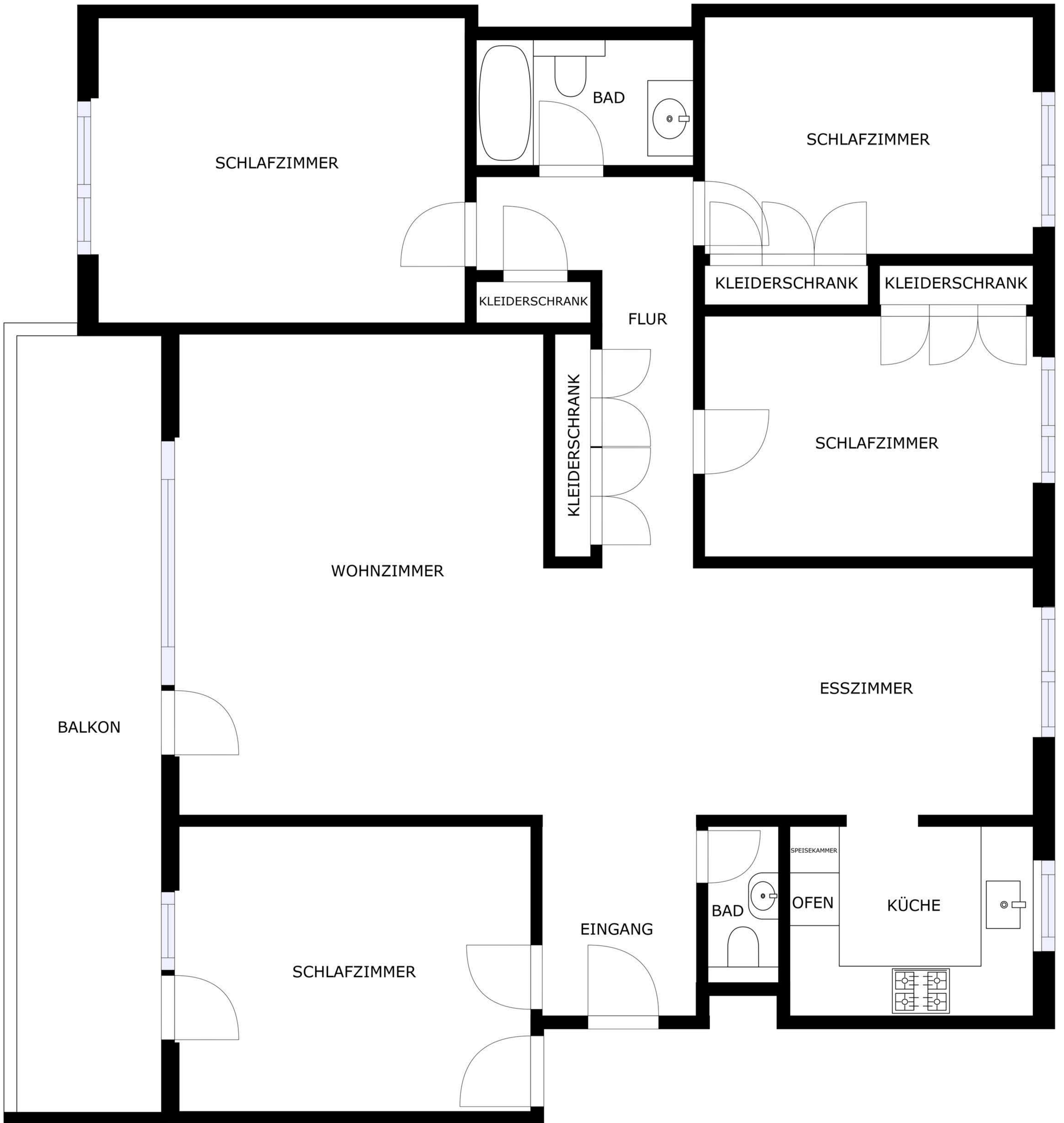
GEBÄUDEPLAN
