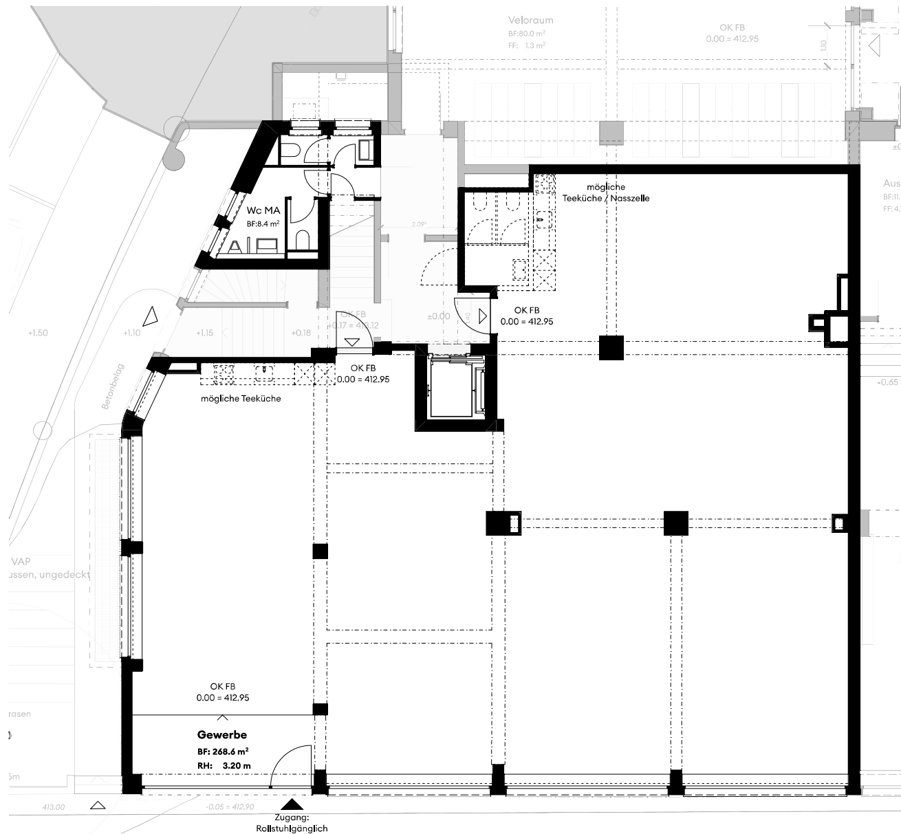
Grundriss 1:100
