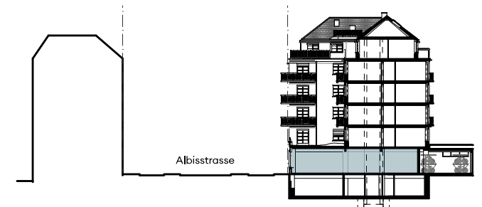
Schnitt 1:500
