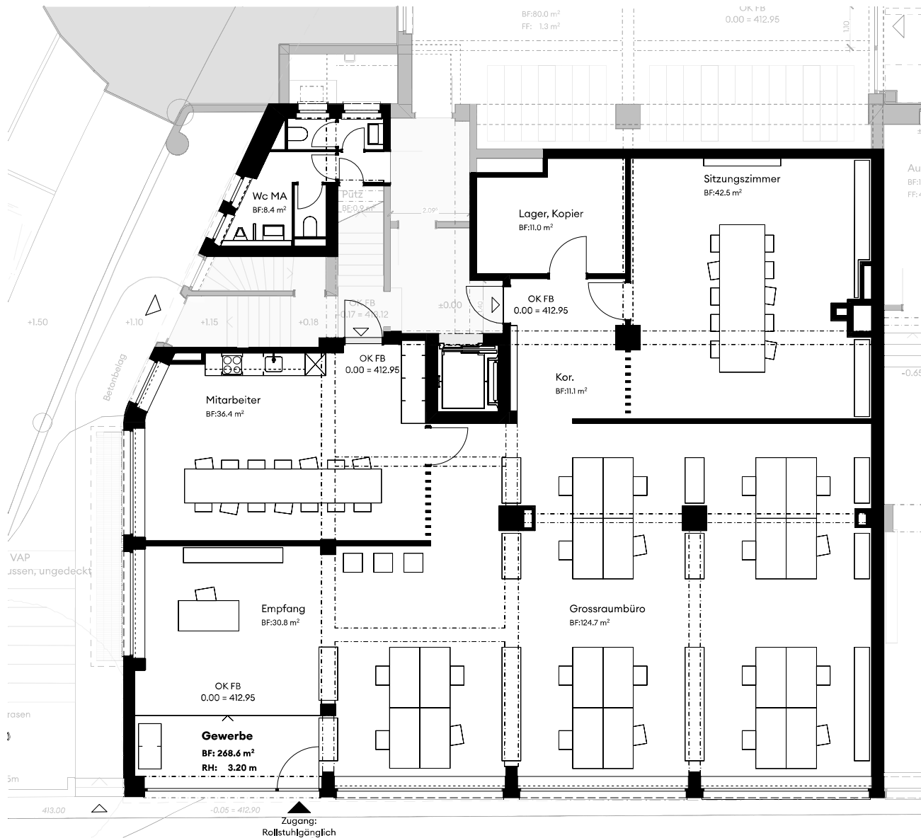
Grundriss 1:100
