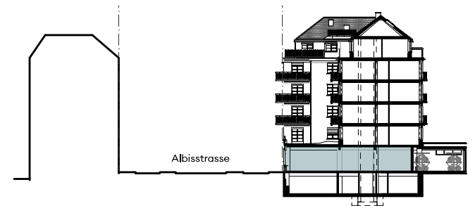
Schnitt 1:500
