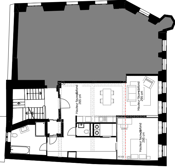
Plan faux-plafonds :
