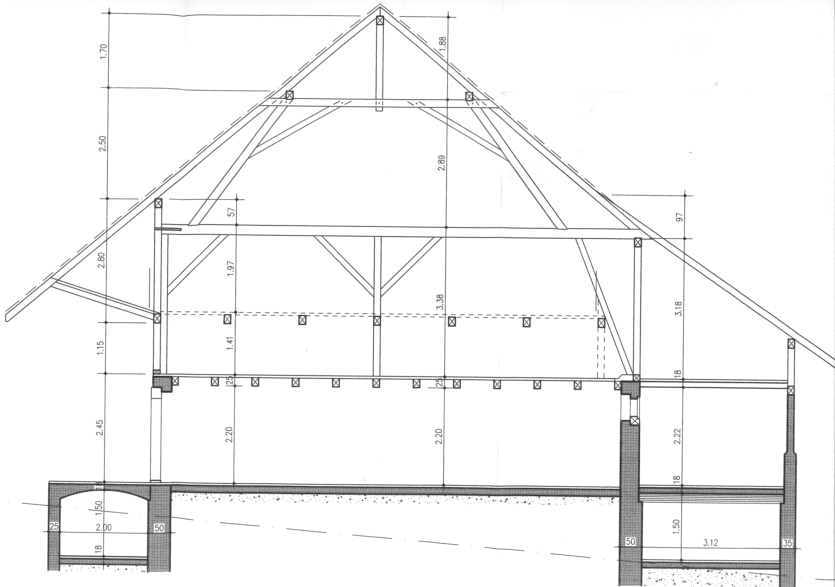
QUERSCHNITT SCHEUNE
