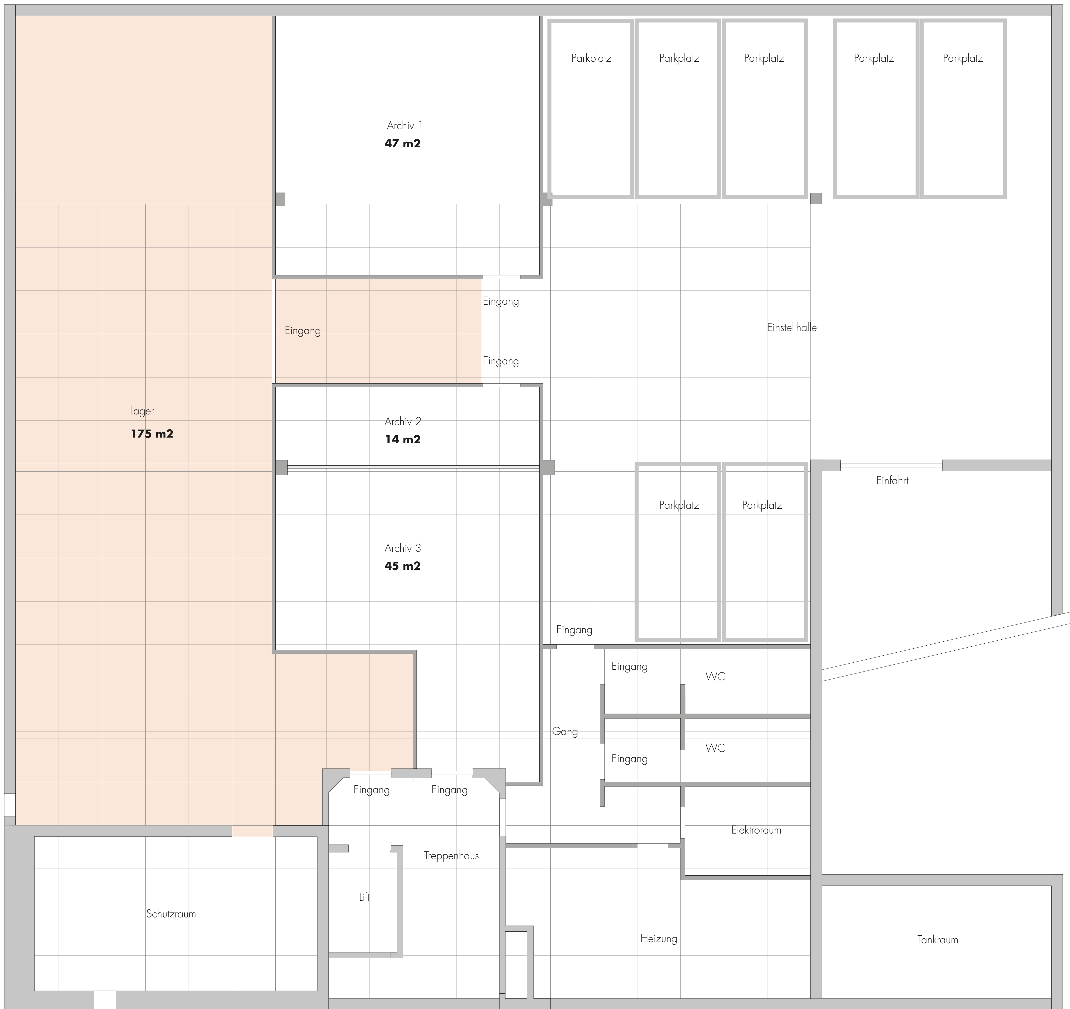
Untergeschoss 1:50
