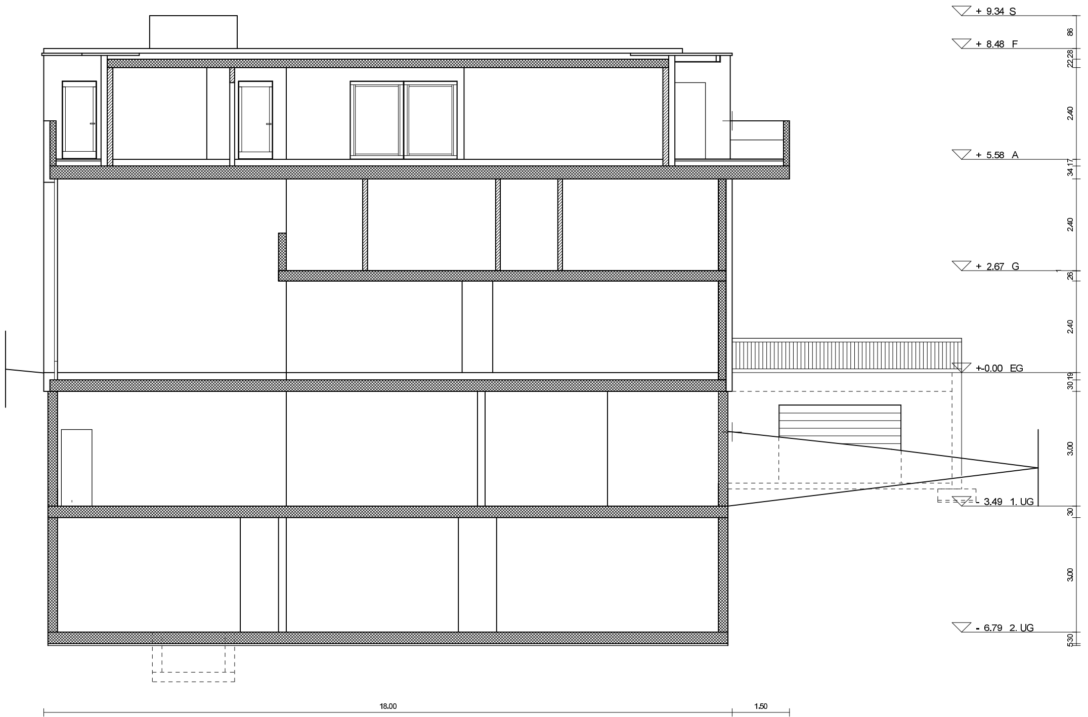
Schnitt A-A
