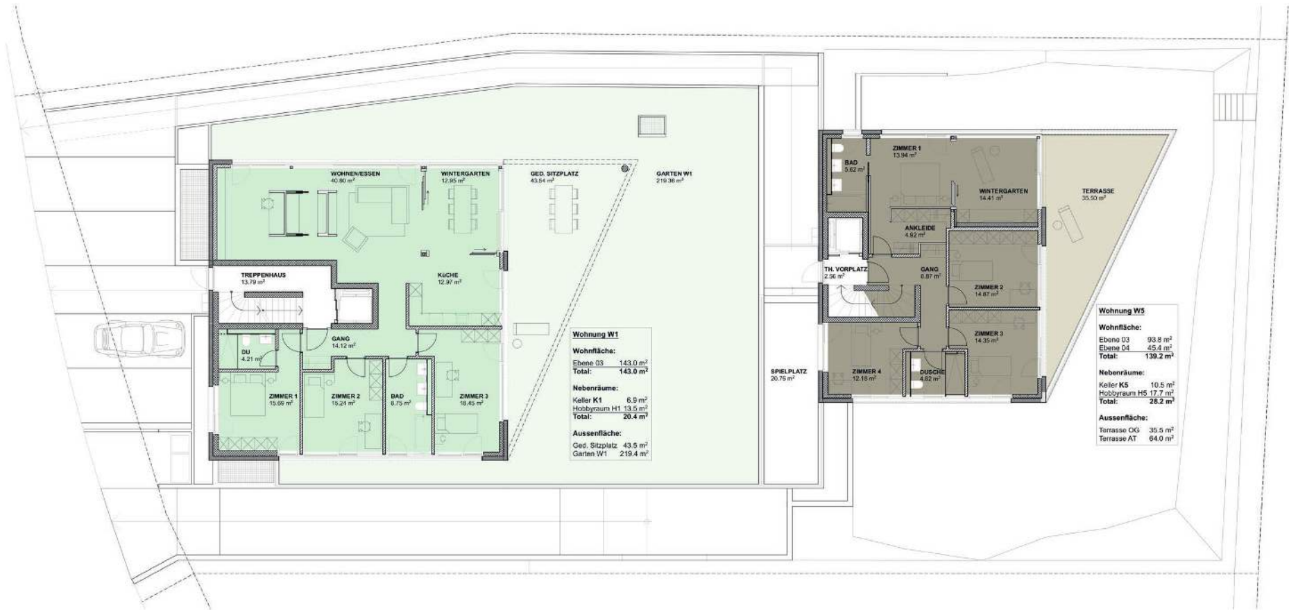
ERDGESCHOSS HAUS A
