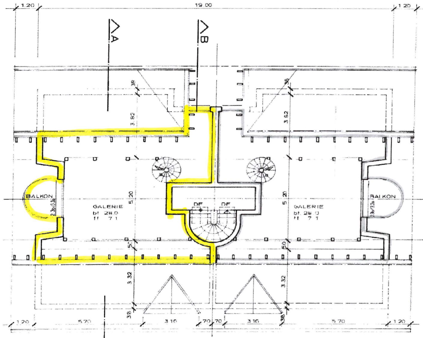
GALERIEGESCHOSS
