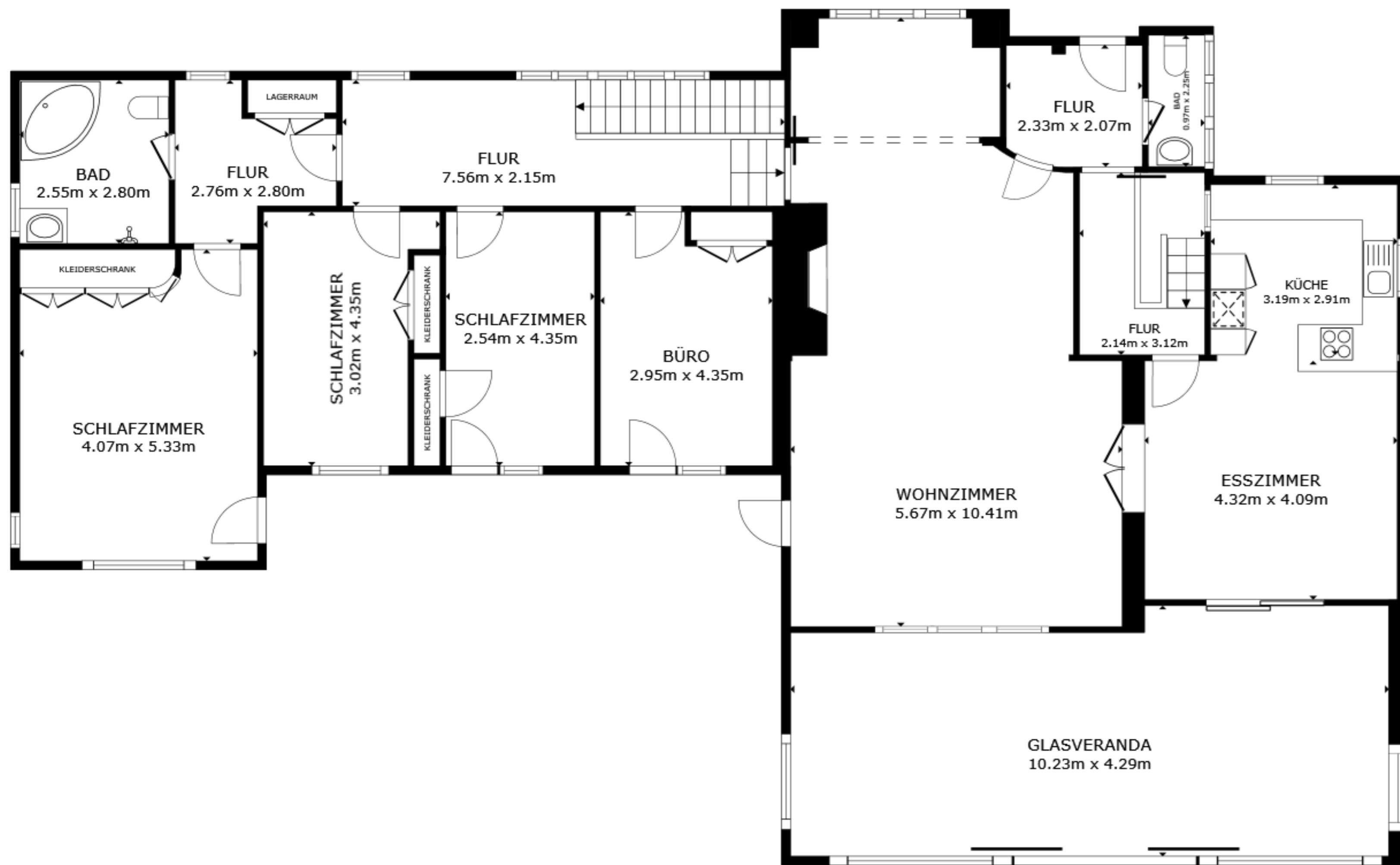
STOCKWERK 3
