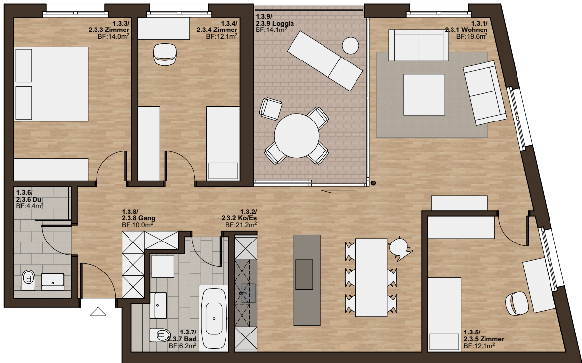
Wohnung 1.3/2.3 4.5-Zi.Whg. NWF:99.6m 2
