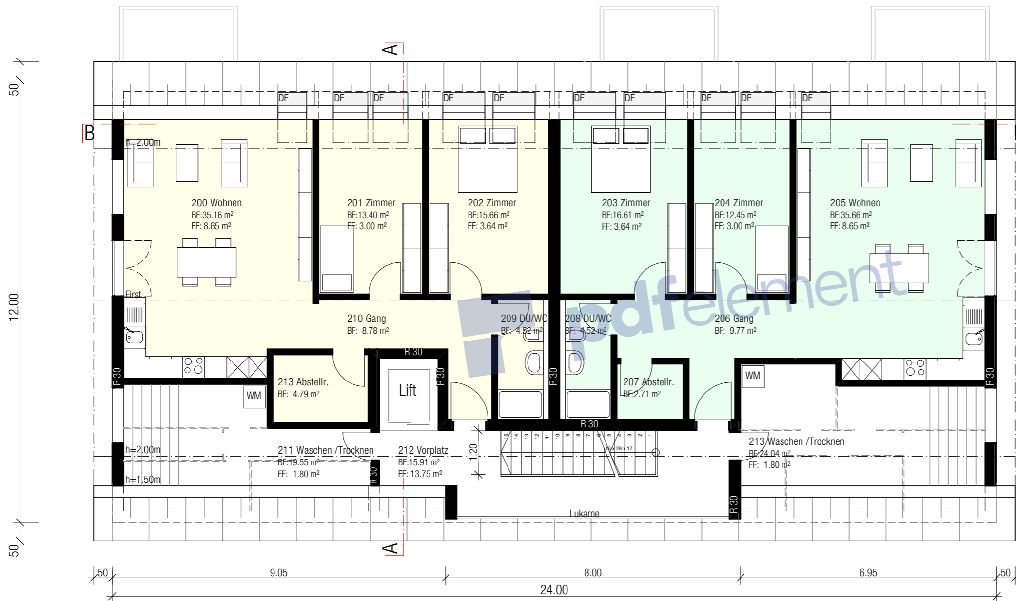
Grundriss Dachgeschoss
