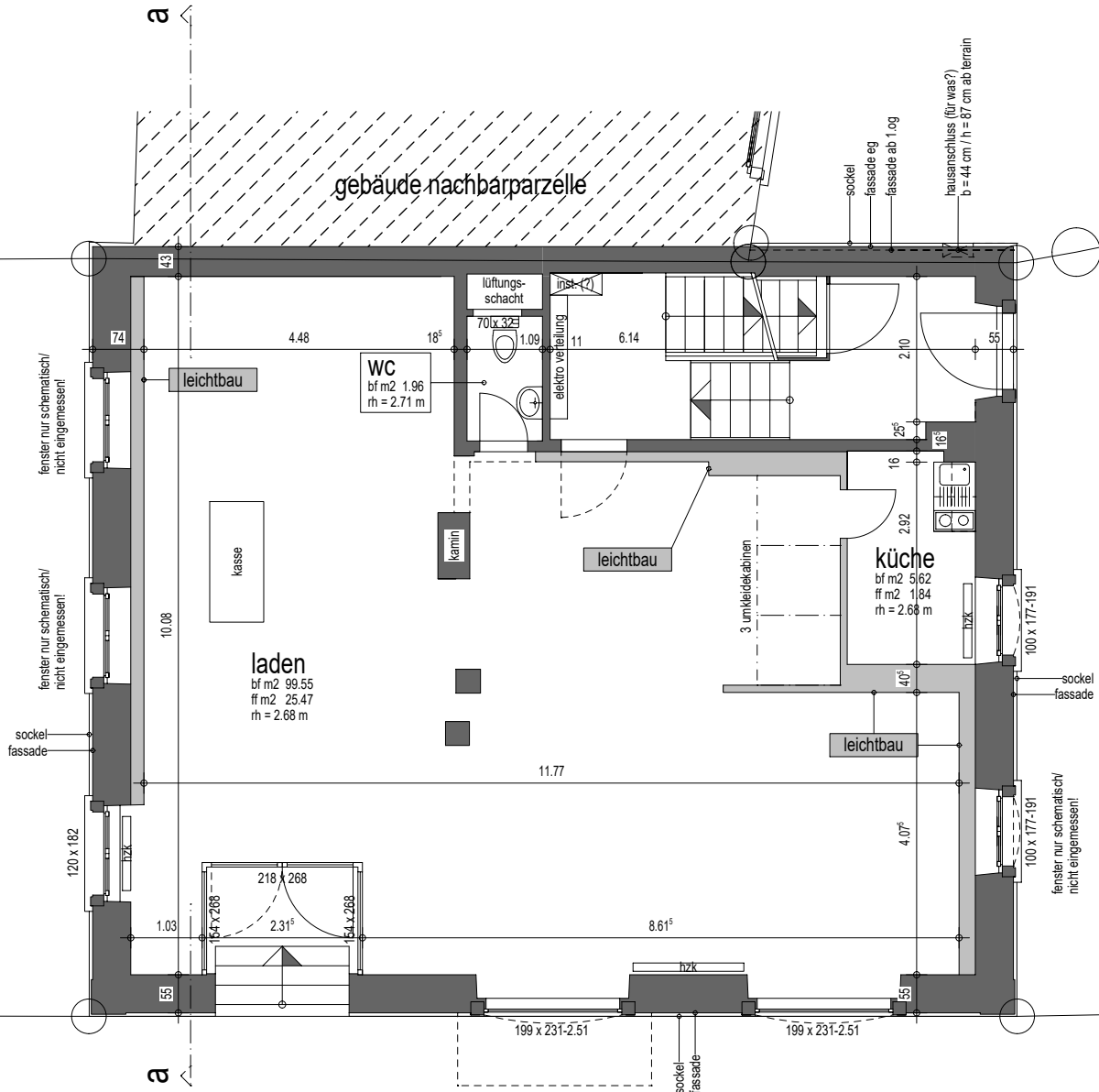
erdgeschoss mst. 1:100
