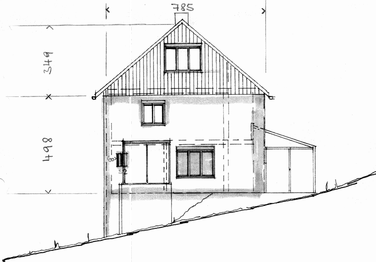
SÜDWESTFASADE
