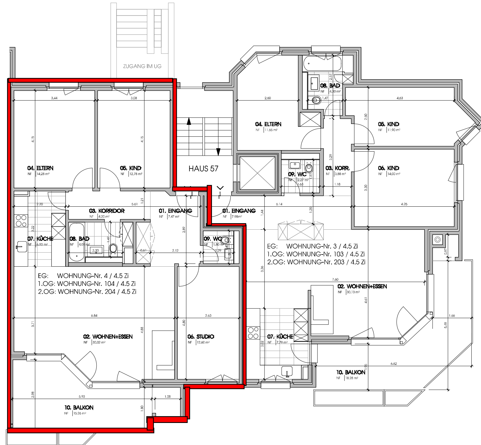
HAUS 57: NORMALGESCHOSS
