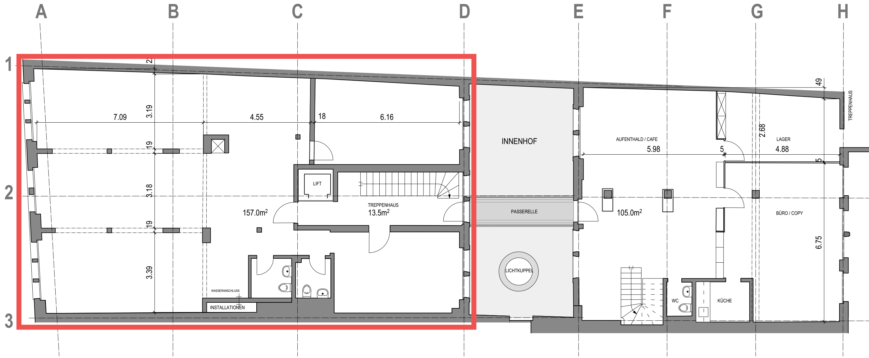
VORDERHAUS 2.OBERGESCHOSS
