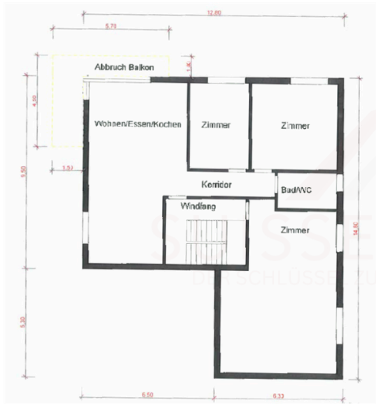
BAUPLAN ERDGESCHOSS
