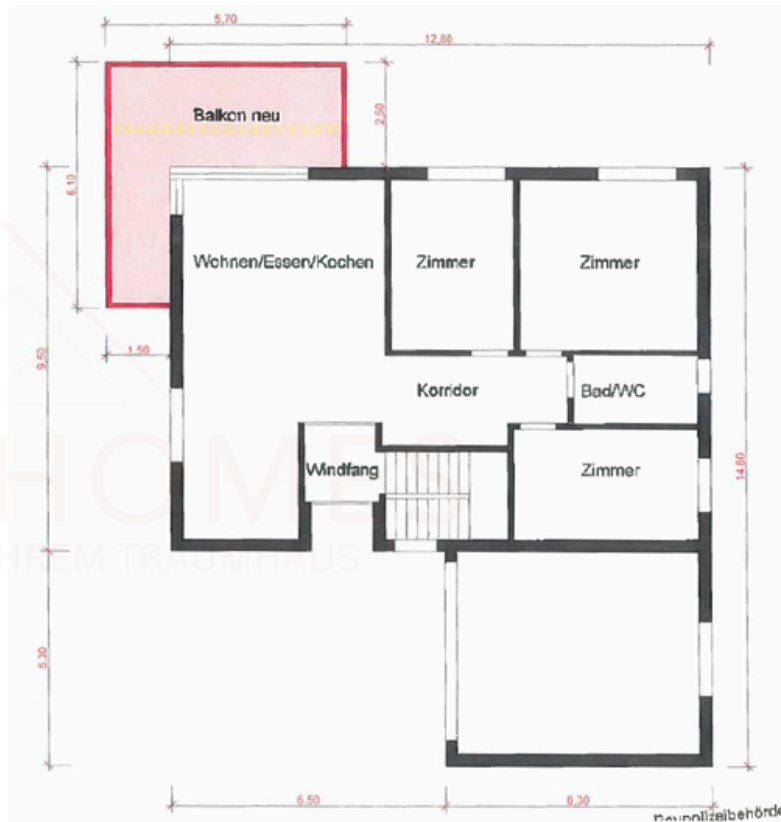
BAUPLAN OBERGESCHOSS
