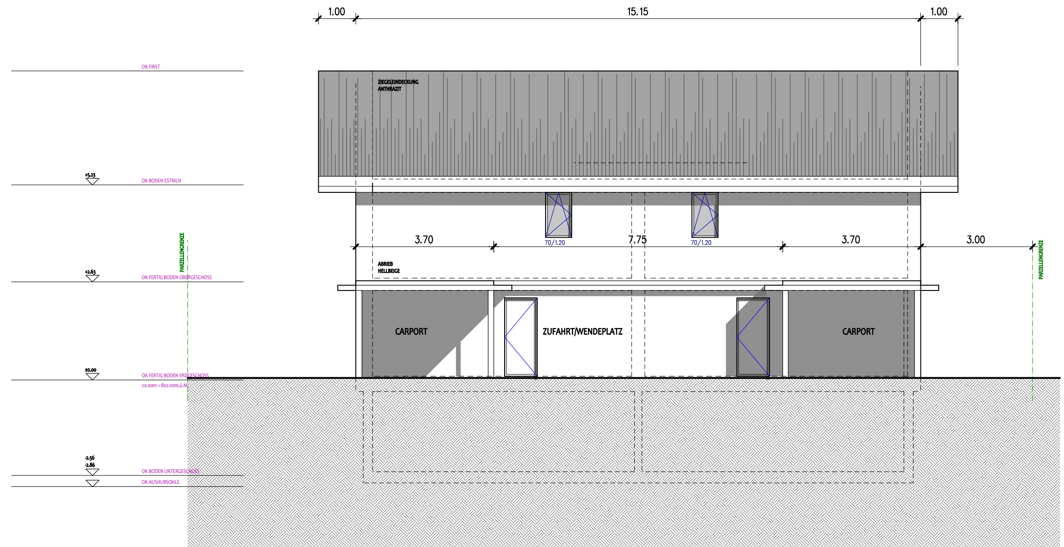
NORDOSTFASSADE
