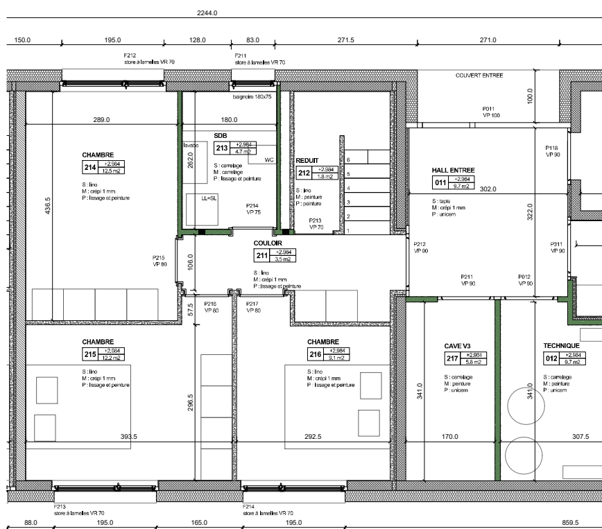
plan étage 1 _ 1:100
