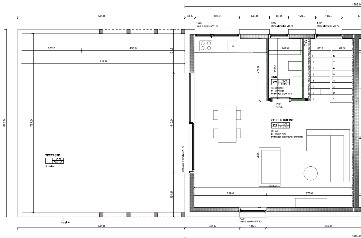
plan Étage 2 _ 1:100
