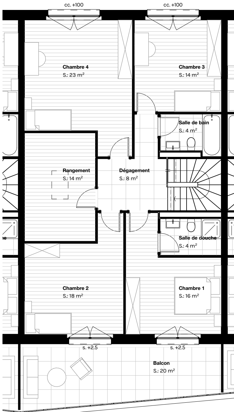
1er étage
