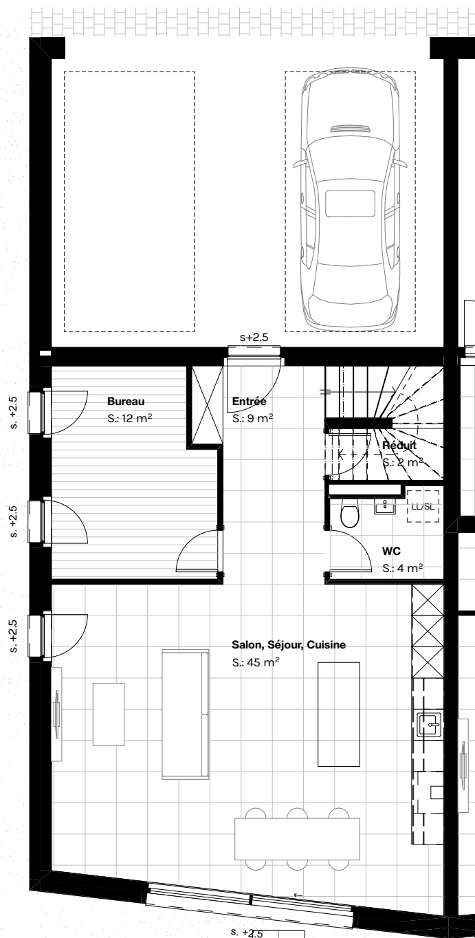
Rez-de-chaussée
