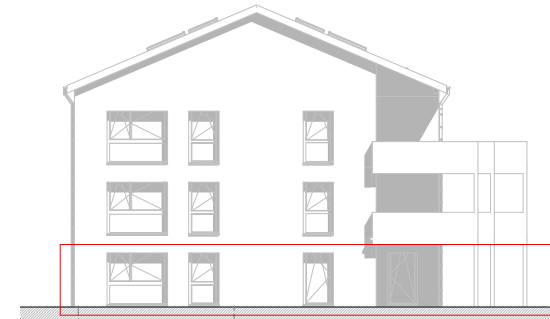
Façade Ouest : 1:200
