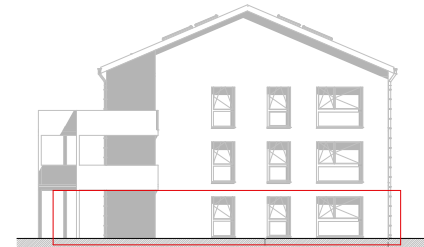
Façade Est : 1:200
