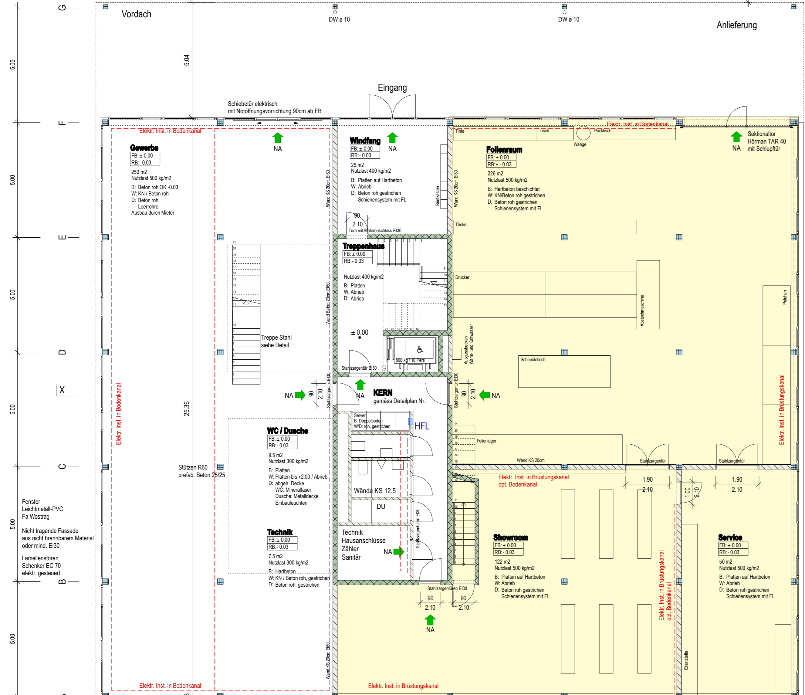
GRUNDRISS ERDGESCHOSS ± 0.00 / 405.00 M. ü. M.
