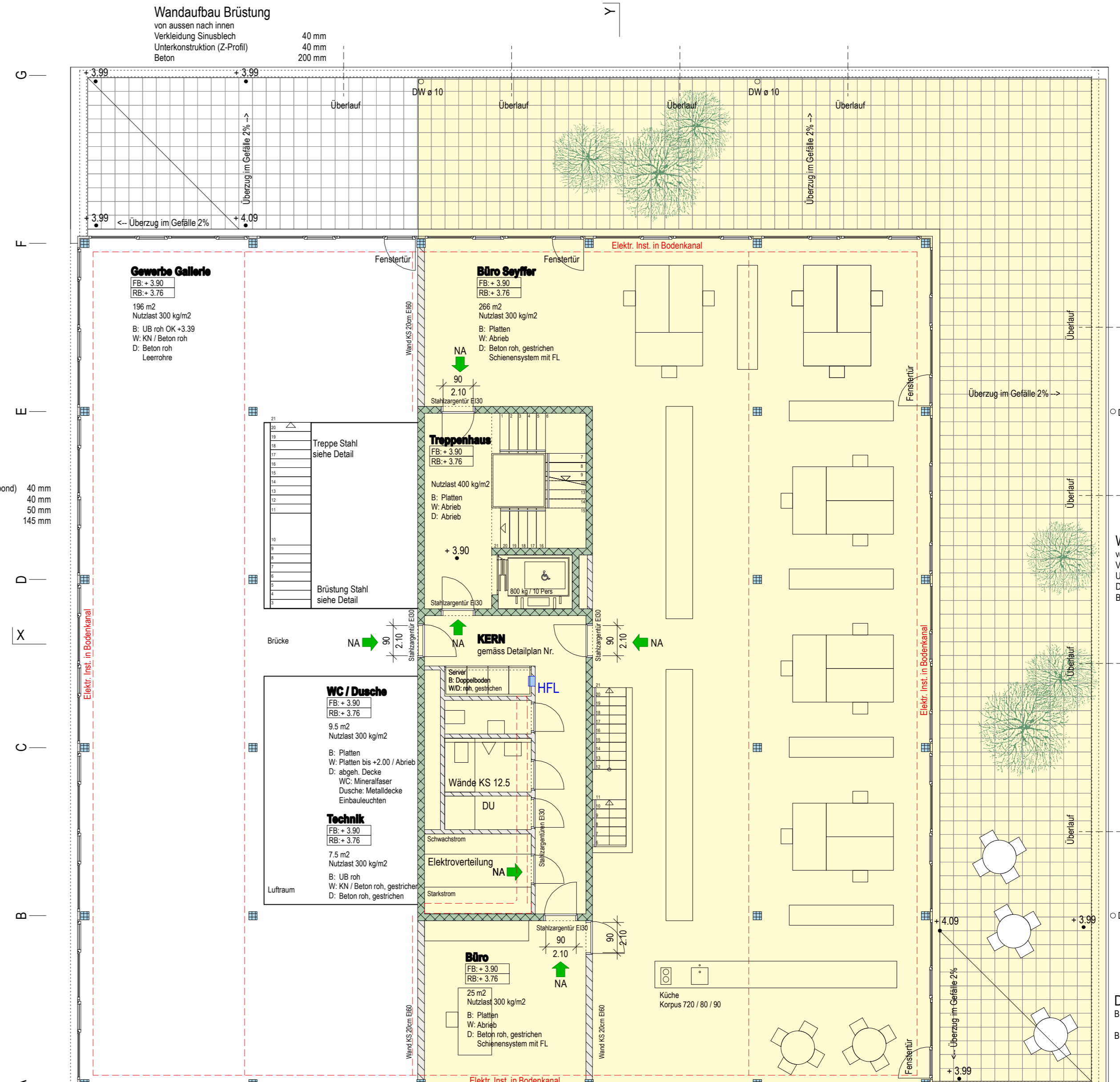
GRUNDRISS 1. OBERGESCHOSS + 3.90 / 408.90 M. ü. M.
