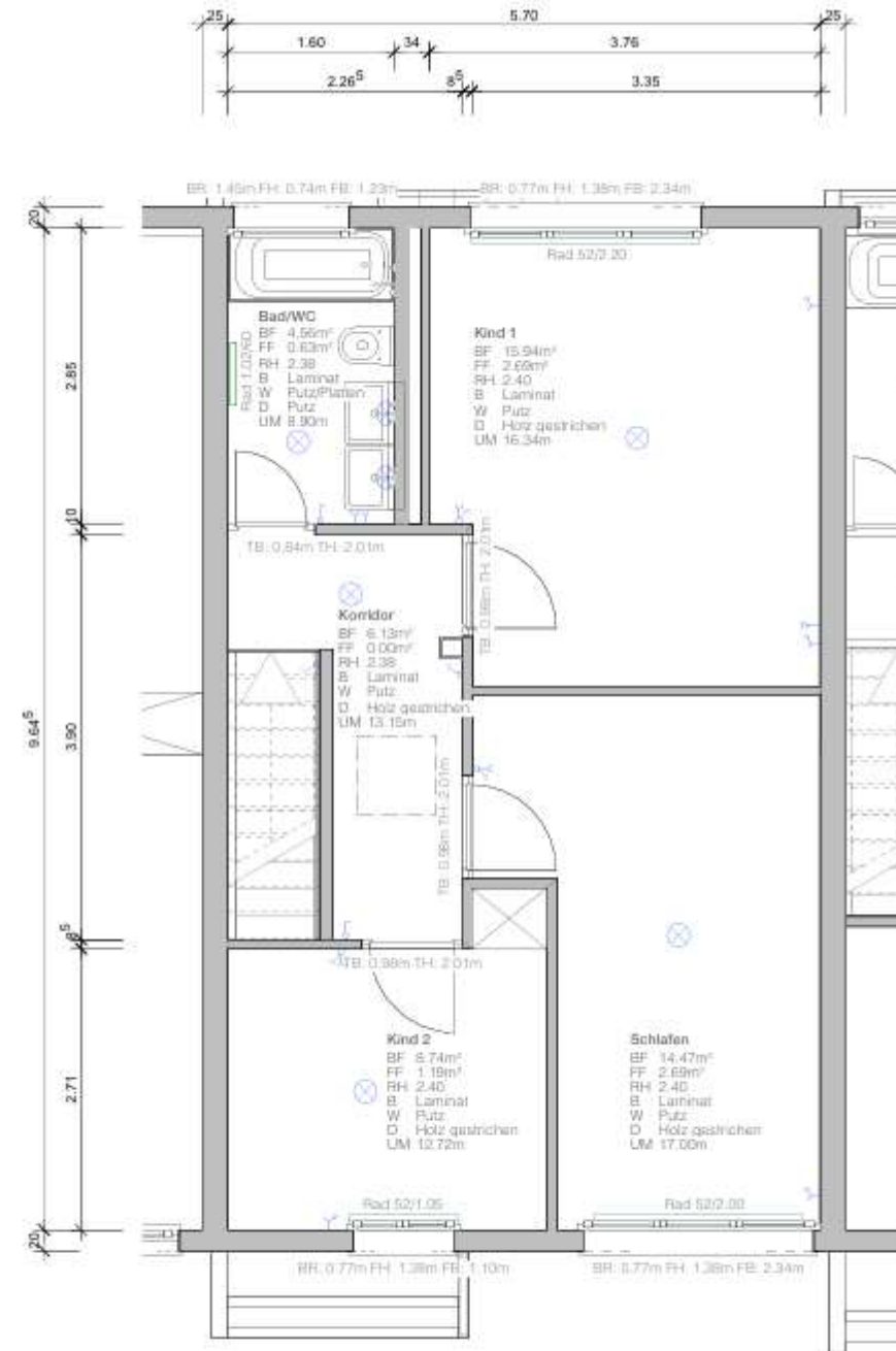
Grundriss OG
