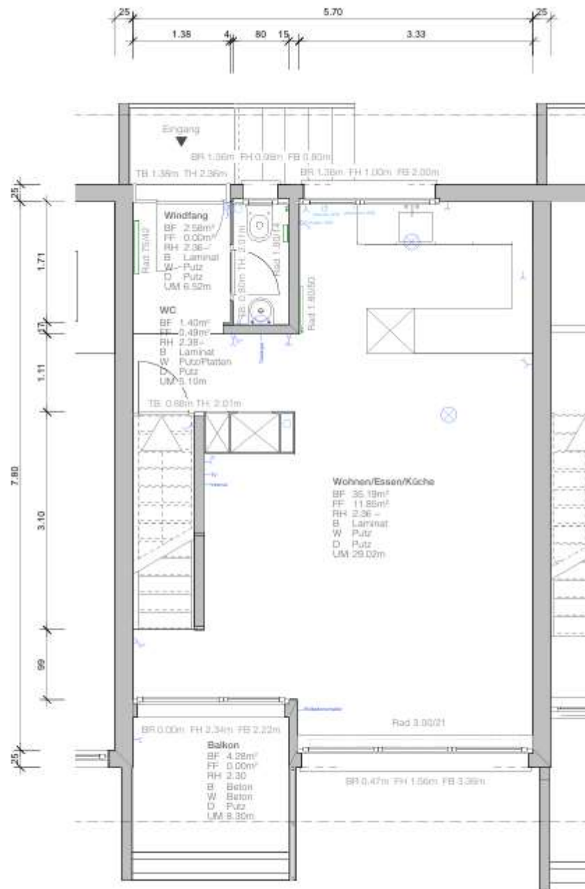
Grundriss EG
