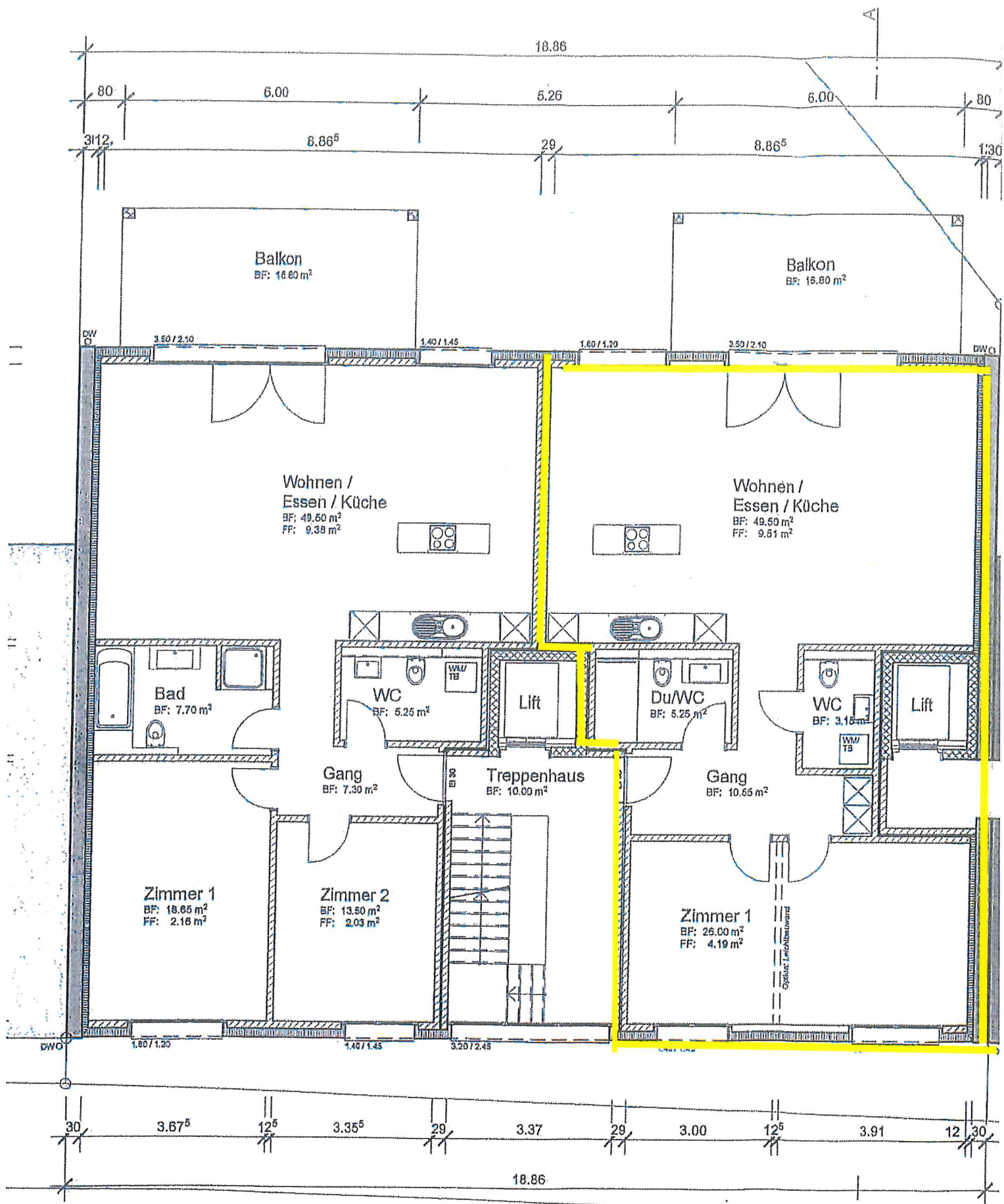
1. - 3. Obergeschoss
