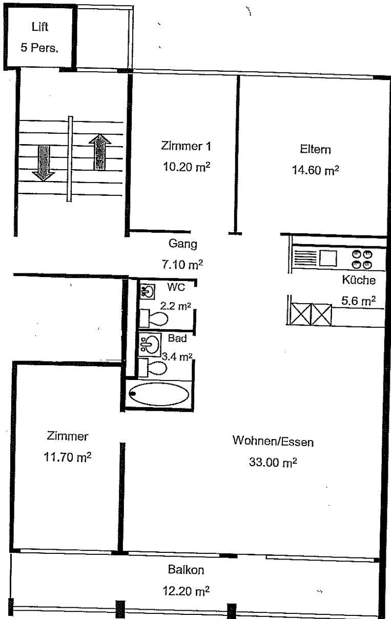
4 1/2 Zimmer-Wohnung
