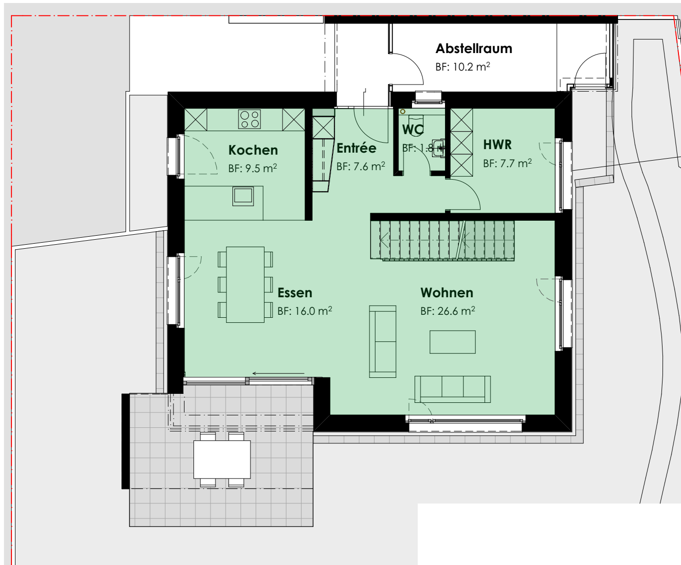
EFH C1 Grundriss Erdgeschoss
