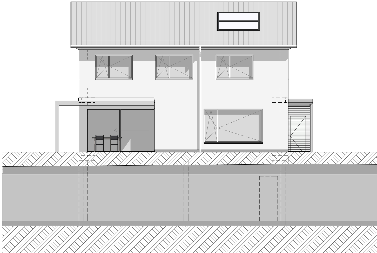
EFH C1 Südwestfassade
