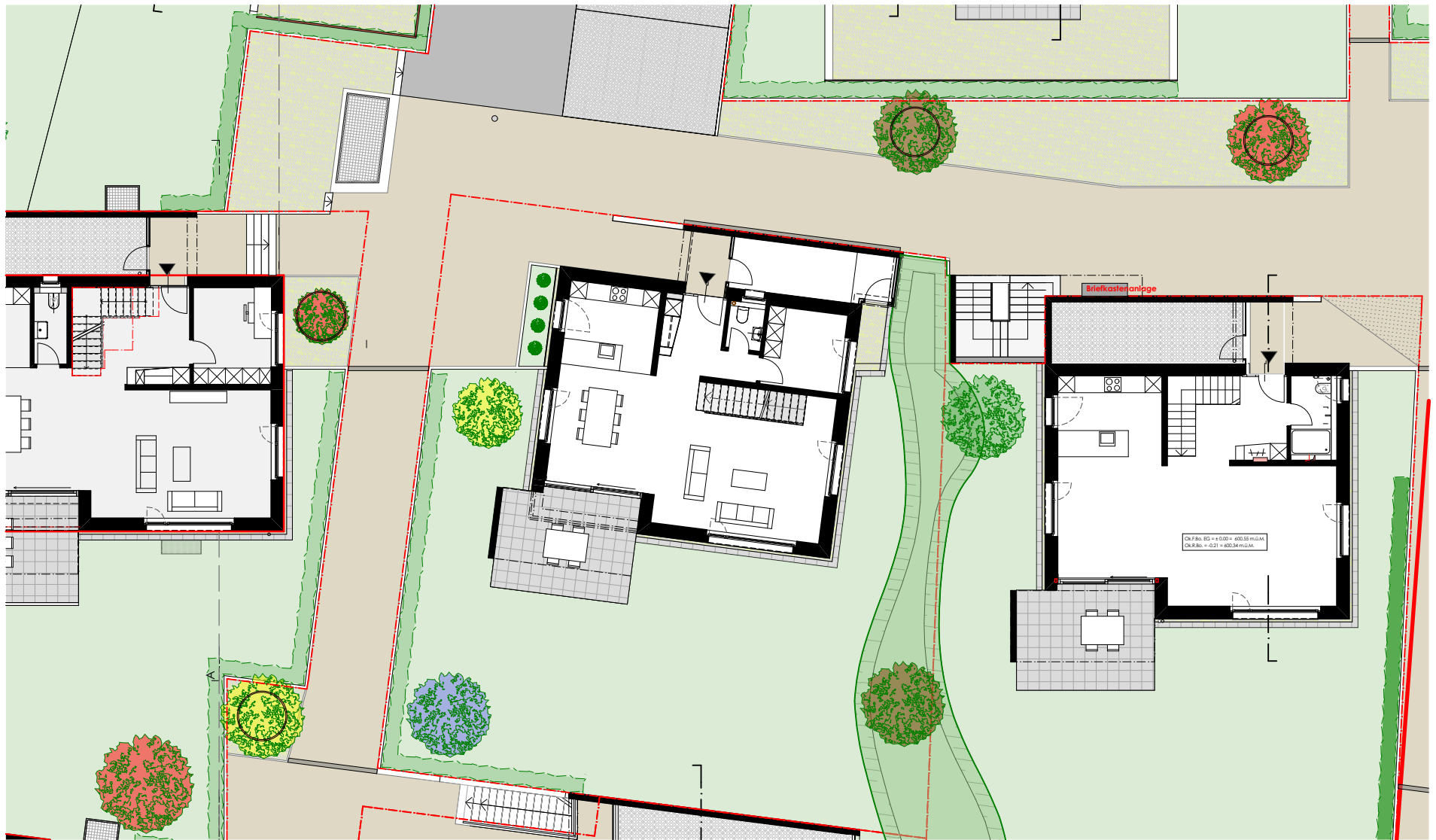
EFH C1 Grundriss EG Umgebung
