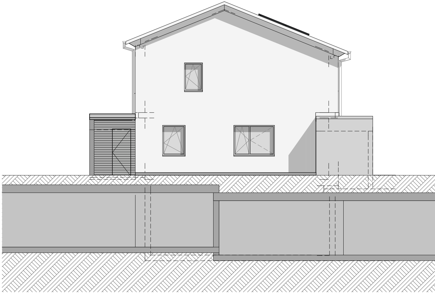
EFH C1 Nordwestfassade
