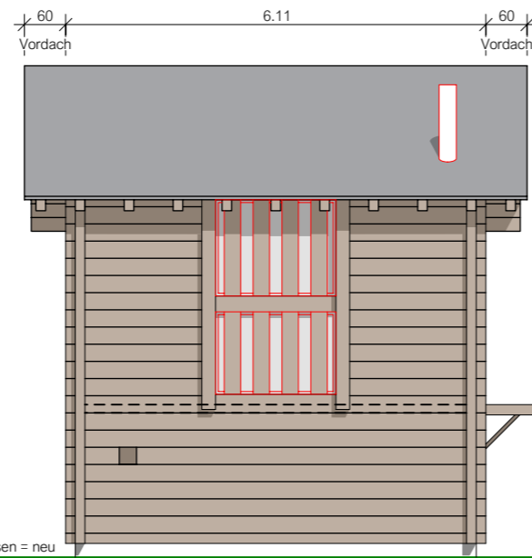
Fassade Süd-Ost
