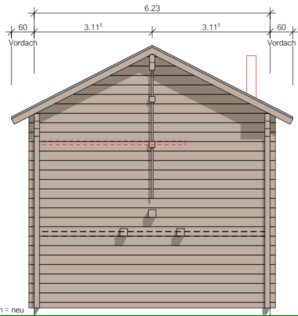
Fassade Süd-West
