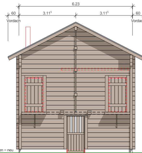
Fassade Nord-Ost
