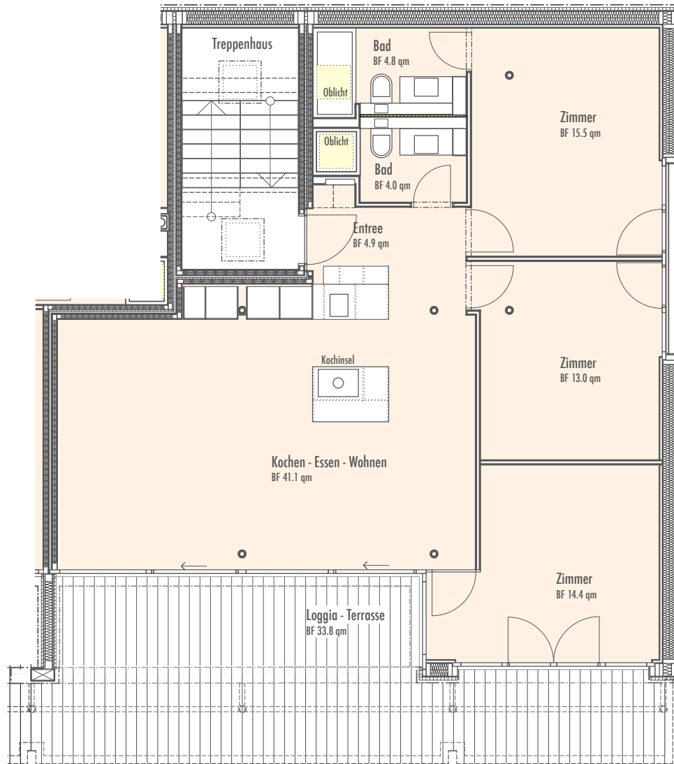
Buchseweg 4 - Attikageschoss - 4.5 Zimmerwohnung links Nettowoohnfläche 99.9 qm; Bruttogeschossfläche 112.7 qm
