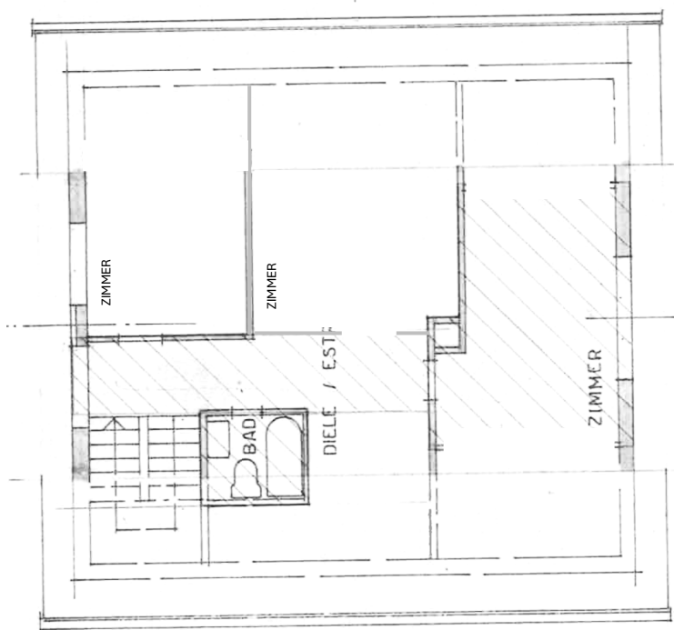
Grundriss Dachgeschoss
