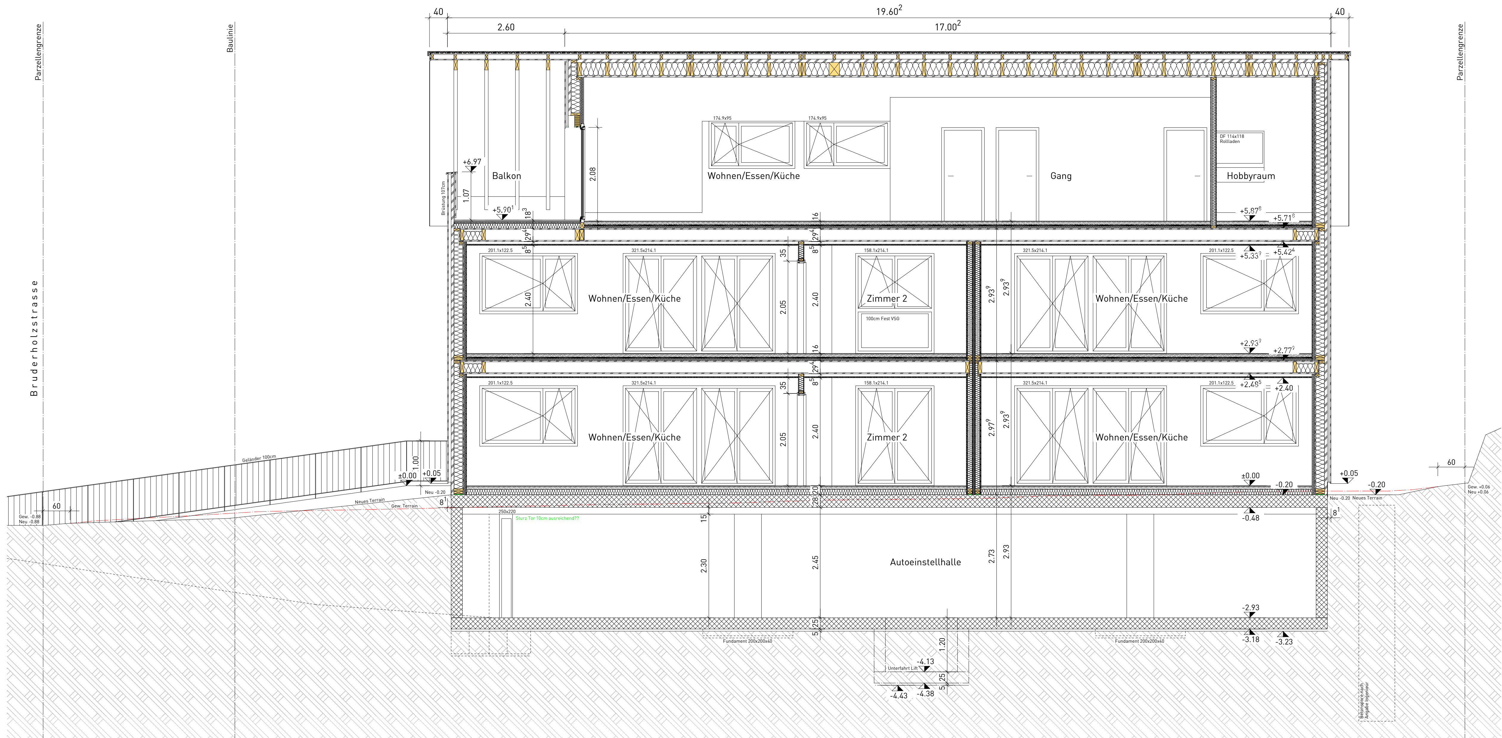
Schnitt A - A
