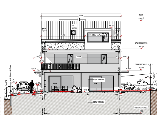
B/1 SÜDEN 1:100
