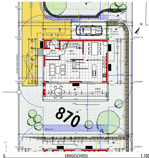
0. ERDGESCHOSS 1:100
