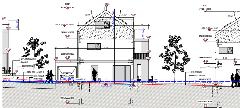
C/4 WESTEN 1:100
