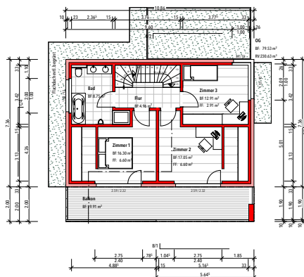
OBERGESCHOSS 1:100
