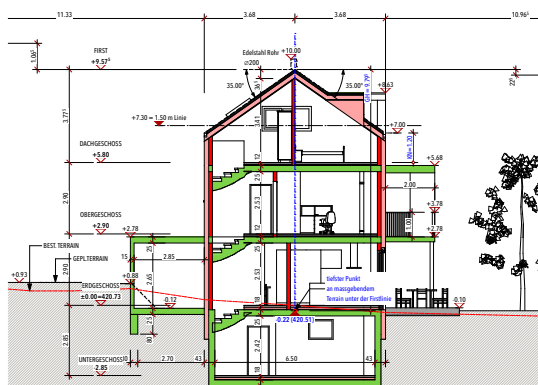
S/1 QUERSCHNITT 1:100
