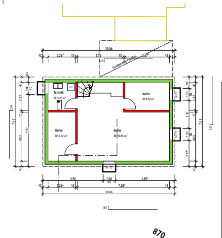
-1. UNTERGESCHOSS 1:100
